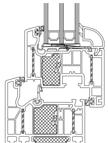
Profieldoorsnede Schüco Alu Inside Coupe de profilé Schüco Alu Inside
